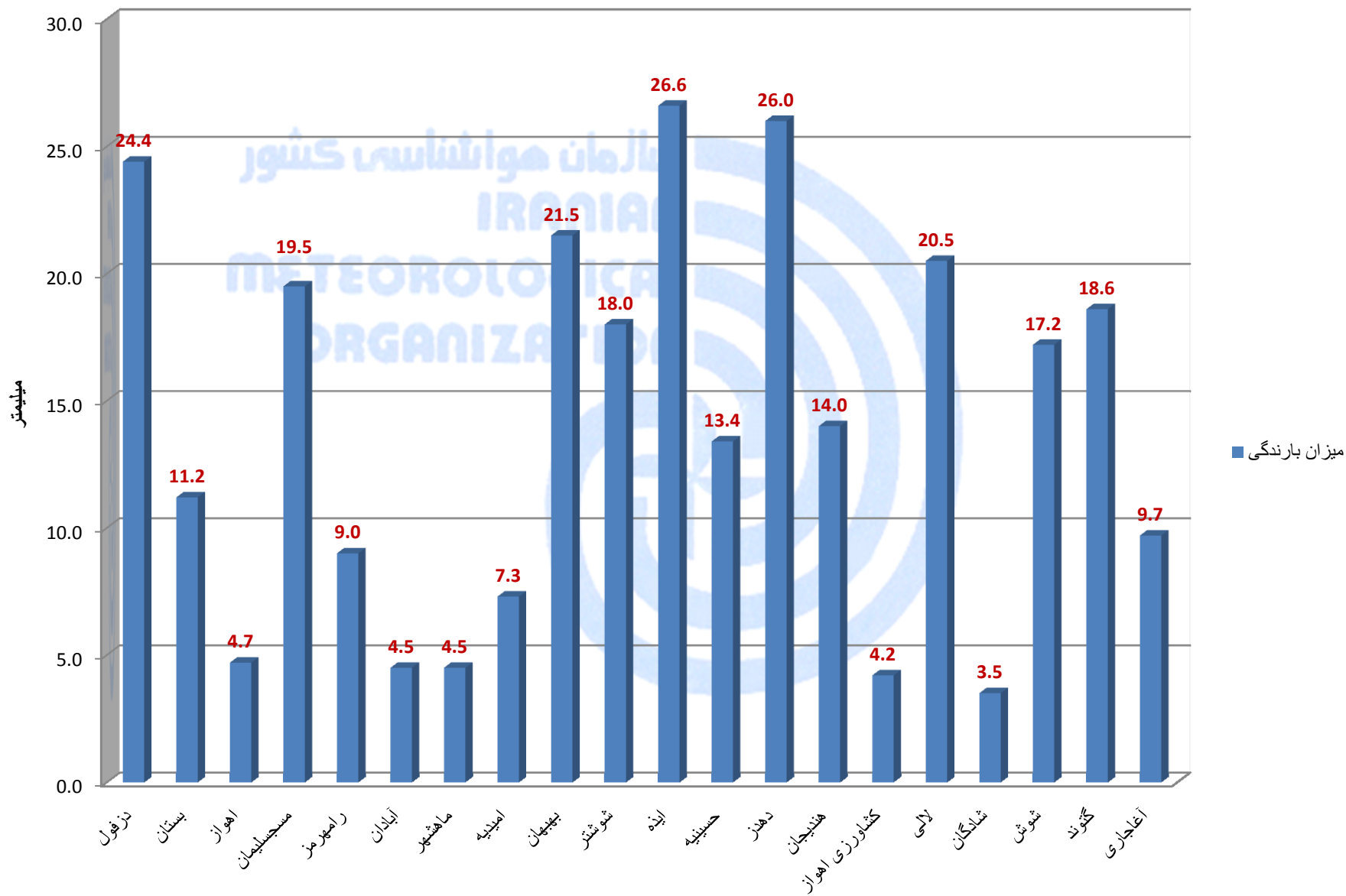
نمودار میزان بارندگی روز ۲۶ دی ۸۹ در استان خوزستان
