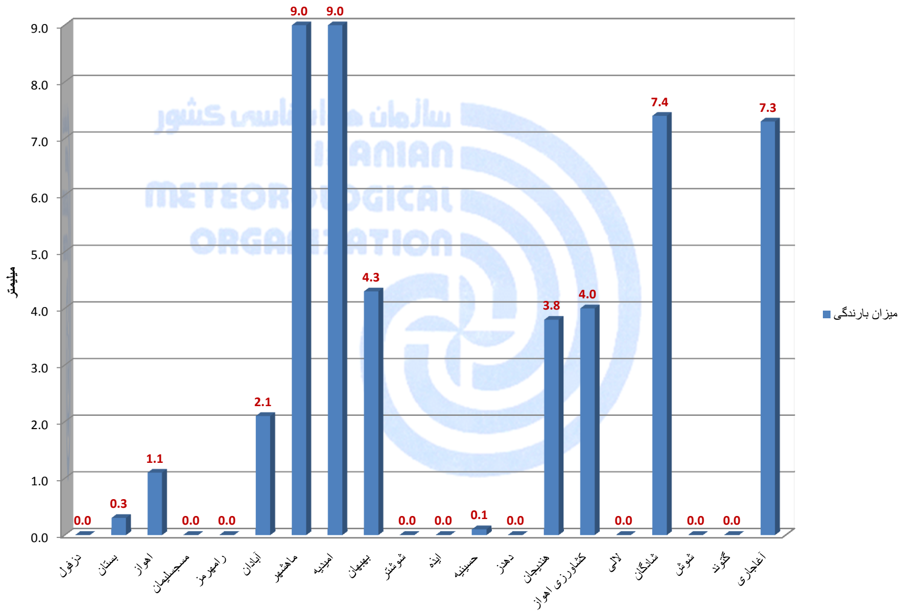
نمودار میزان بارندگی روز ۱۹ بهمن ۸۹ در استان خوزستان
