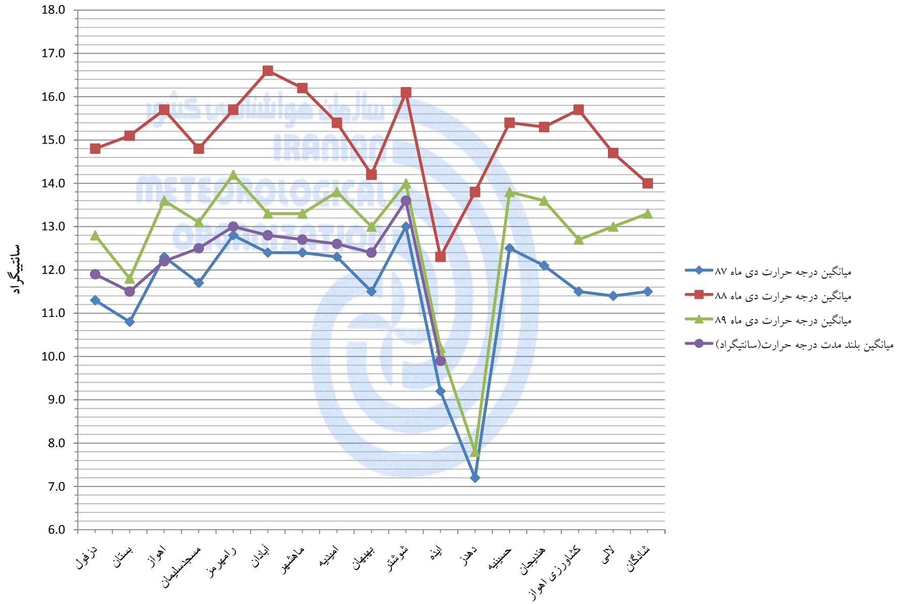
نوسانات میانگین دمای هوا دی ماه ۸۹ ایستگاههای استان خوزستان و مقایسه با سالهای گذشته و بلند مدت آن
